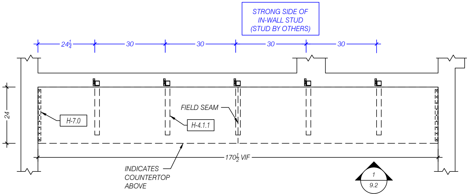
2 PLAN - AV COORDINATION ROOM 126 SCALE 1:24 (1/2"=1'-0") ARCH REF: 15/AE408
